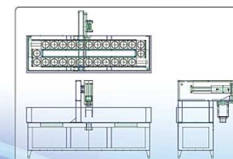
染杯供應系統 (Cup Feeder)
